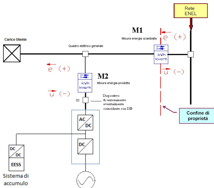
Figura H-3.4.a) Schema di collegamento dei sistemi di misura e-distribuzione presso un punto di prelievo di un Produttore BT e MT ( \leq 20\text{kW} ) con sistema di accumulo nella parte in c.c. dell'impianto a valle del sistema di misura dell'energia prodotta.
